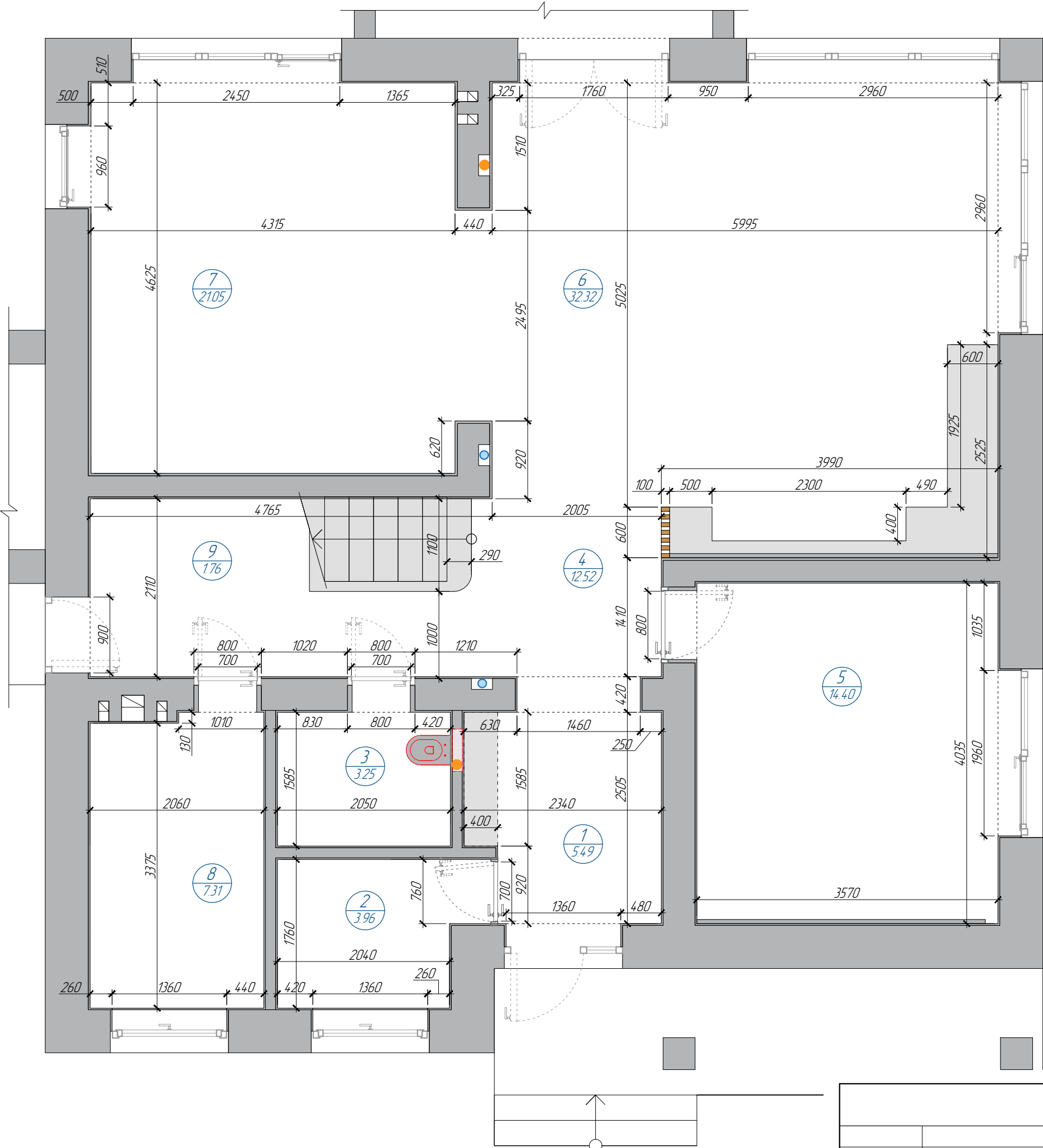
План 1 этажа
