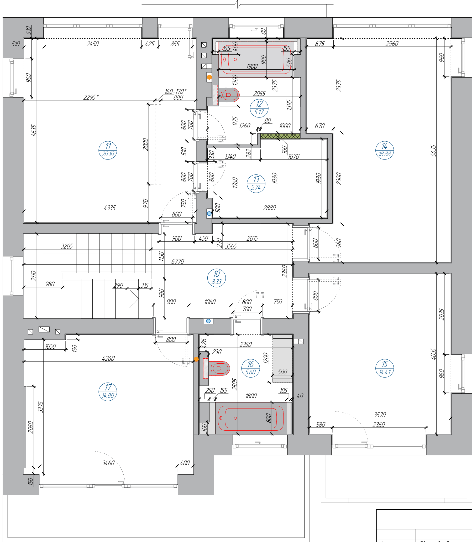
План 2 этажа
